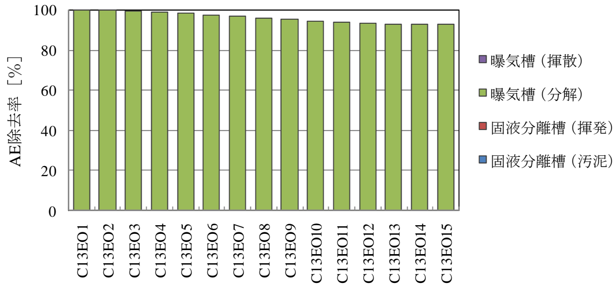
図IV.9 下水処理場における AE の工程別除去率 (6-box モデル, C13)
