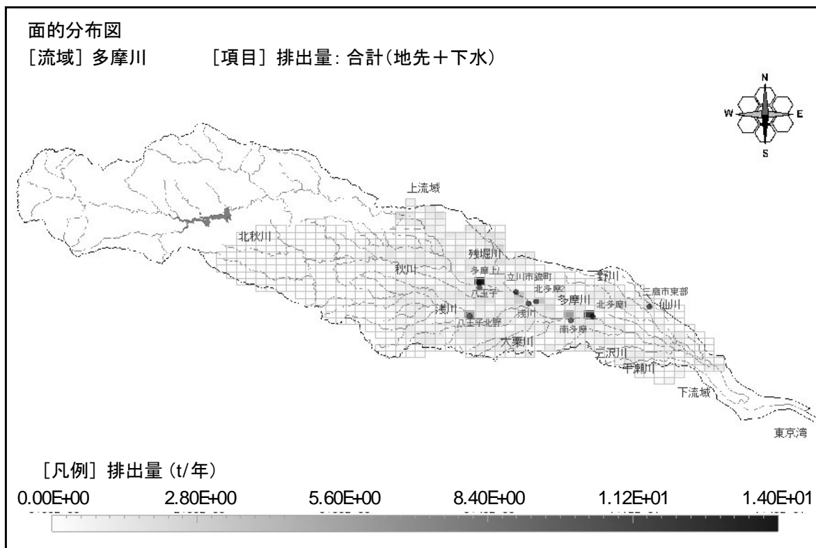
図VI.7 多摩川流域における排出量の分布 (流通量ベース)
