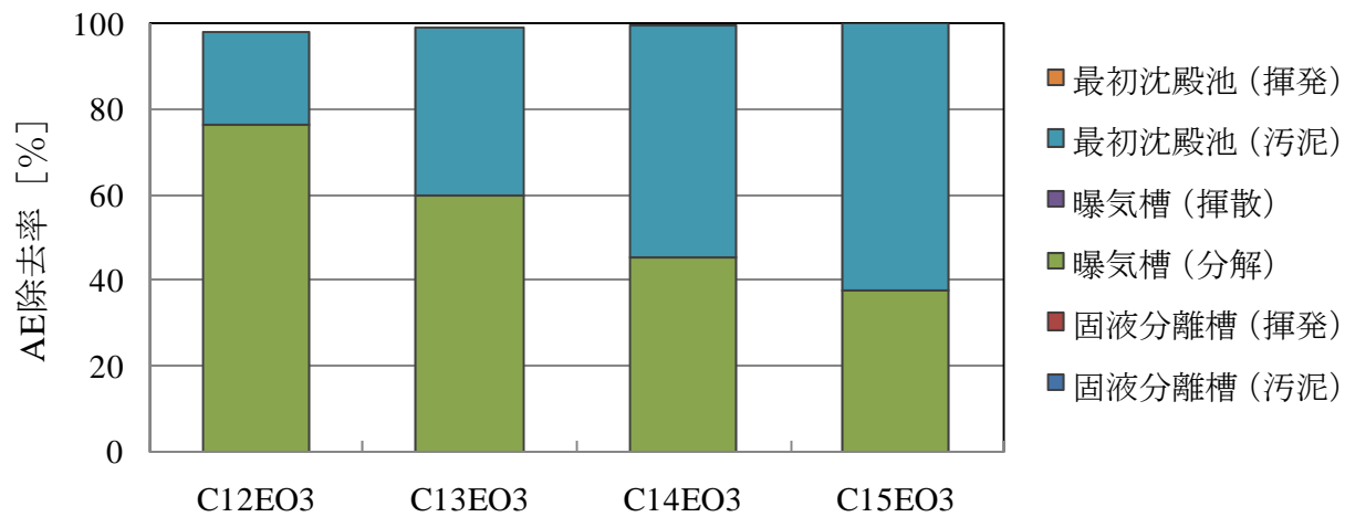
図IV.7 下水処理場における AE の工程別除去率 (9-box モデル, EO3)
